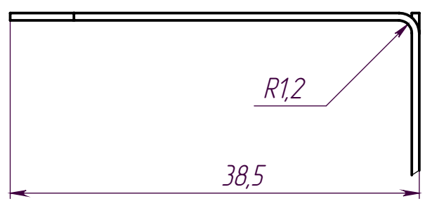
А (2 : 1) 4 места
