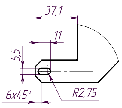
Б (1 : 2) 4 места
